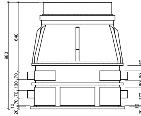
ELEVATION B
