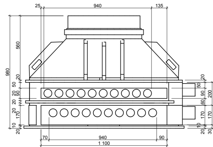
ELEVATION A
